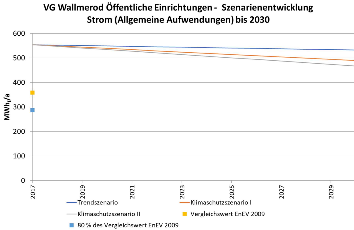
Abbildung 4-8 Entwicklung Endenergieverbrauch Strom Kommunale Einrichtungen VG Wallmerod
