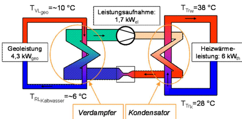
Abbildung 6-6 Schema Kompressionswärmepumpe
