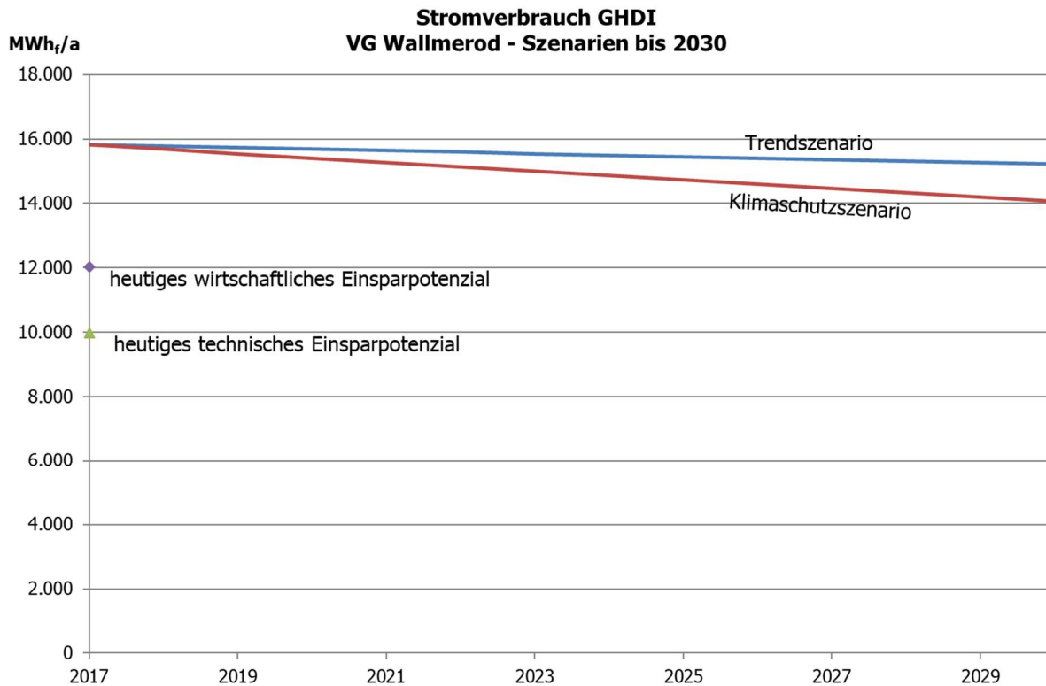
Abbildung 4-12 Entwicklung Endenergieverbrauch Strom Sektor GHDI VG Wallmerod
