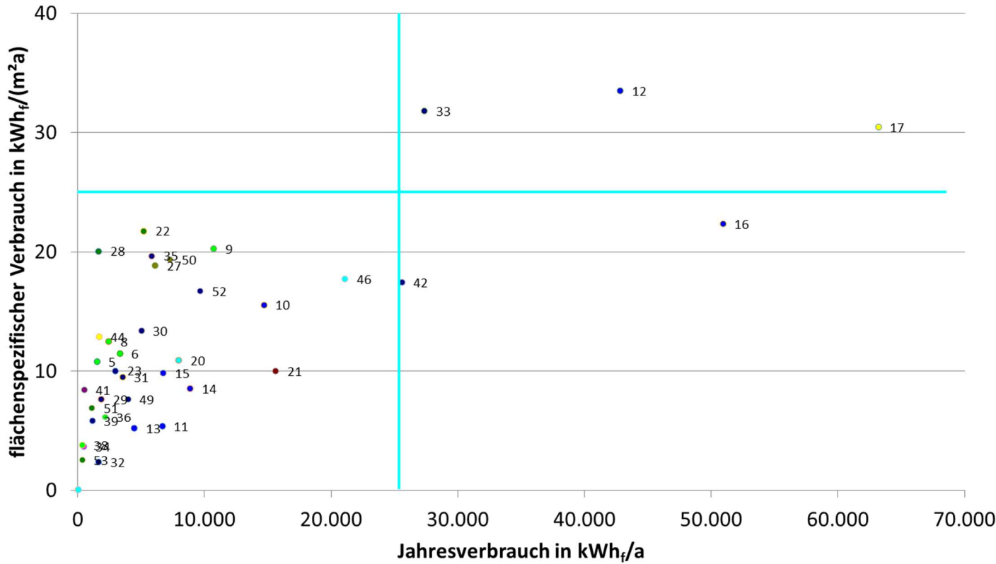
Abbildung 3-11 Auswertung Endenergieverbrauch Strom der kommunalen Liegenschaften in der Verbandsgemeinde Wallmerod (Ausschnitt II)
