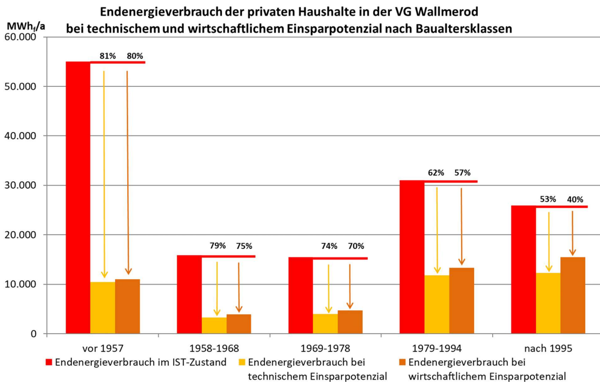
Abbildung 4-2 Einsparpotenzial Wärme in Private Haushalte nach Baualtersklassen VG Wallmerod
