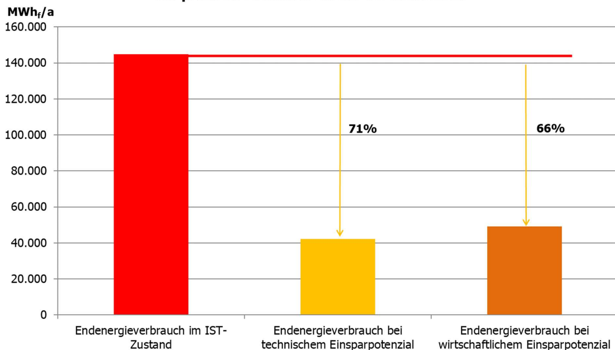
Abbildung 4-1 Einsparpotenzial Wärme in Private Haushalte VG Wallmerod
