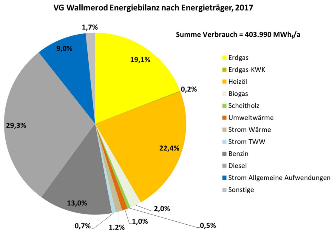
Abbildung 3-3 Gesamtendenergieverbrauch nach Energieträger – VG Wallmerod – Bilanzjahr 2017
