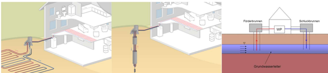
Abbildung 6-4 Erdwärmekollektoranlage, Erdwärmesonde und Erdwärmenutzung mittels Grundwasser
