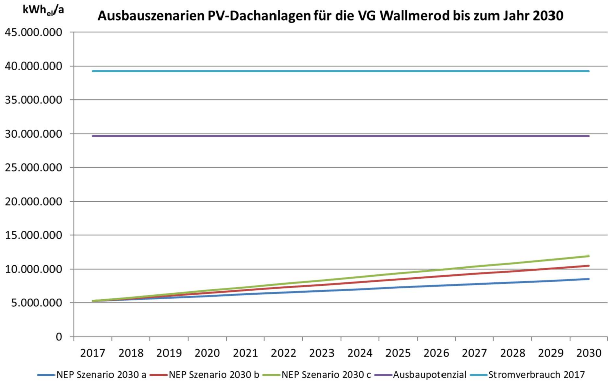
Abbildung 6-2 Ausbauszenarien PV-Dachflächen (Ertrag) für die Verbandsgemeinde Wallmerod
