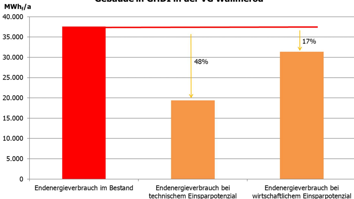
Abbildung 4-9 Technisches und wirtschaftliches Einsparpotenzial Sektor GHDI VG Wallmerod
