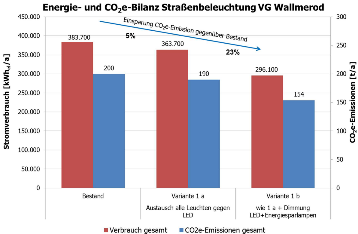
Abbildung 4-14: Energie- und CO 2 e-Bilanz Straßenbeleuchtung VG Wallmerod
