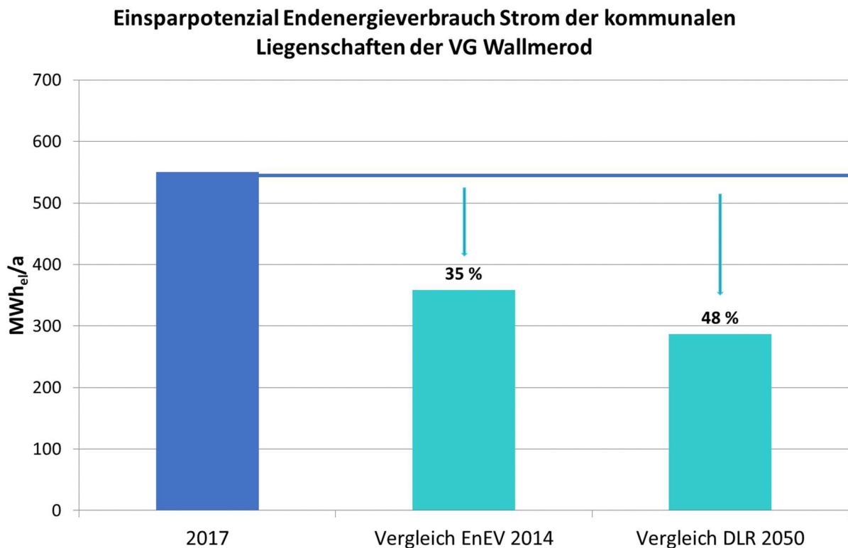
Abbildung 4-7 Endenergieeinsparpotenzial zur Stromversorgung Kommunale Einrichtungen VG Wallmerod
