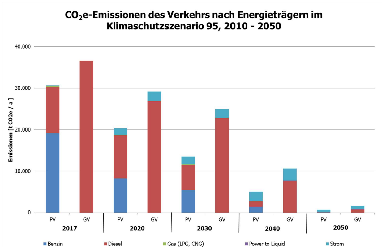
Abbildung 5-6 CO 2 e-Emissionen des Personen- und Güterverkehr nach Energieträgern im Klimaschutzscenario 95, 2010 – 2050
