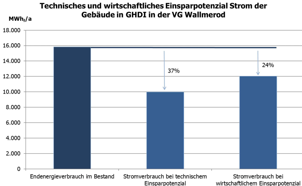
Abbildung 4-11 Technisches und wirtschaftliches Einsparpotenzial Strom Sektor GHDI VG Wallmerod
