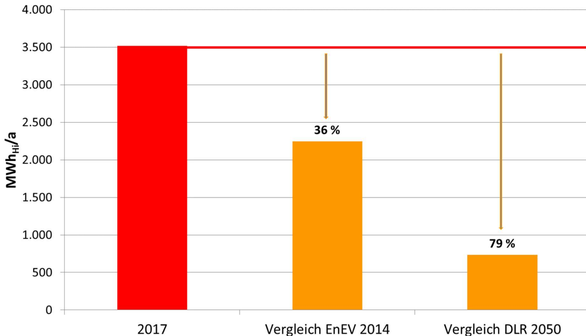
Abbildung 4-5 Endenergieeinsparpotenzial Wärmeversorgung Kommunale Einrichtungen VG Wallmerod
