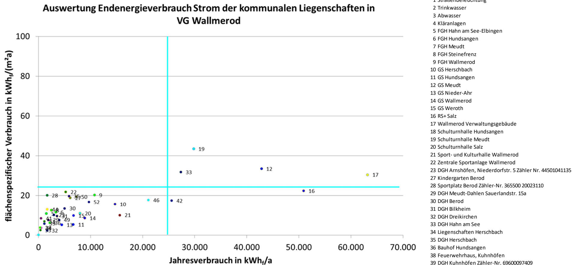
Abbildung 3-10 Auswertung Endenergieverbrauch Strom der kommunalen Liegenschaften in der Verbandsgemeinde Wallmerod
